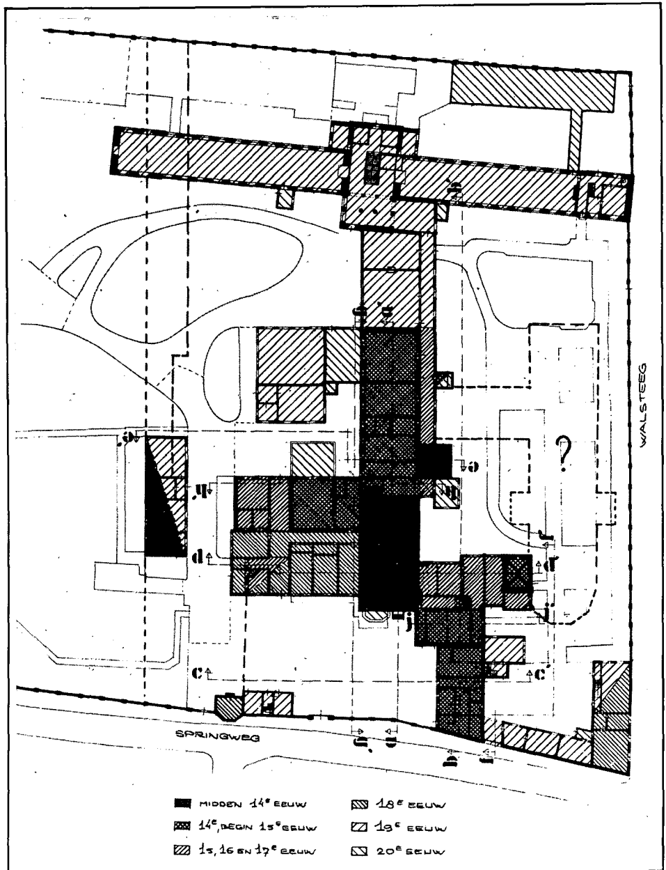
Het Duitse Huis; plattegrond met globale periodisering. De verdwenen oude gedeelten zijn gestippeld weergegeven.
