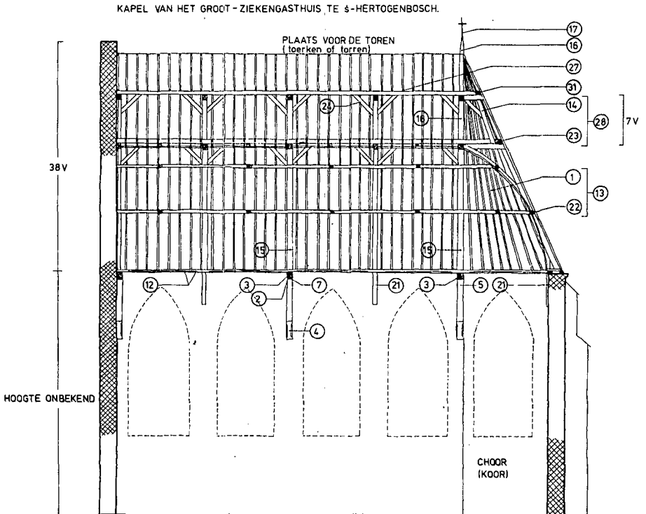
REKONSTRUKTIE LANGSDOORSNEDE VOLGENS EEN BESTEK UIT 1487
