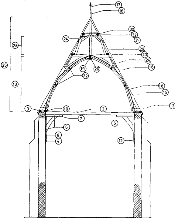
REKONSTRUKTIE DWARSDOORSNEDE VOLGENS EEN BESTEK UIT 1487.
