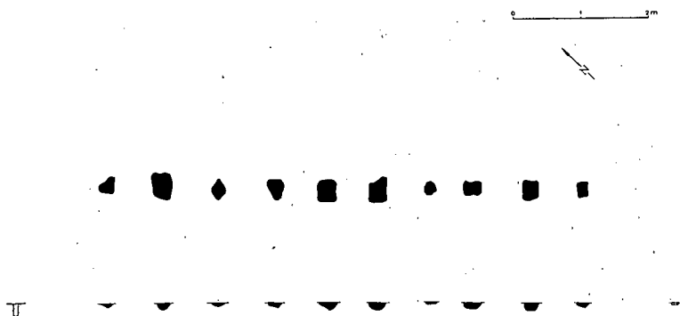
Nuenen, De Collsche Hoeve. Plattegrond van paalkuilen en doorsneden. Vermoedelijk uit de Romeinse tijd. Schaal 1:100.
