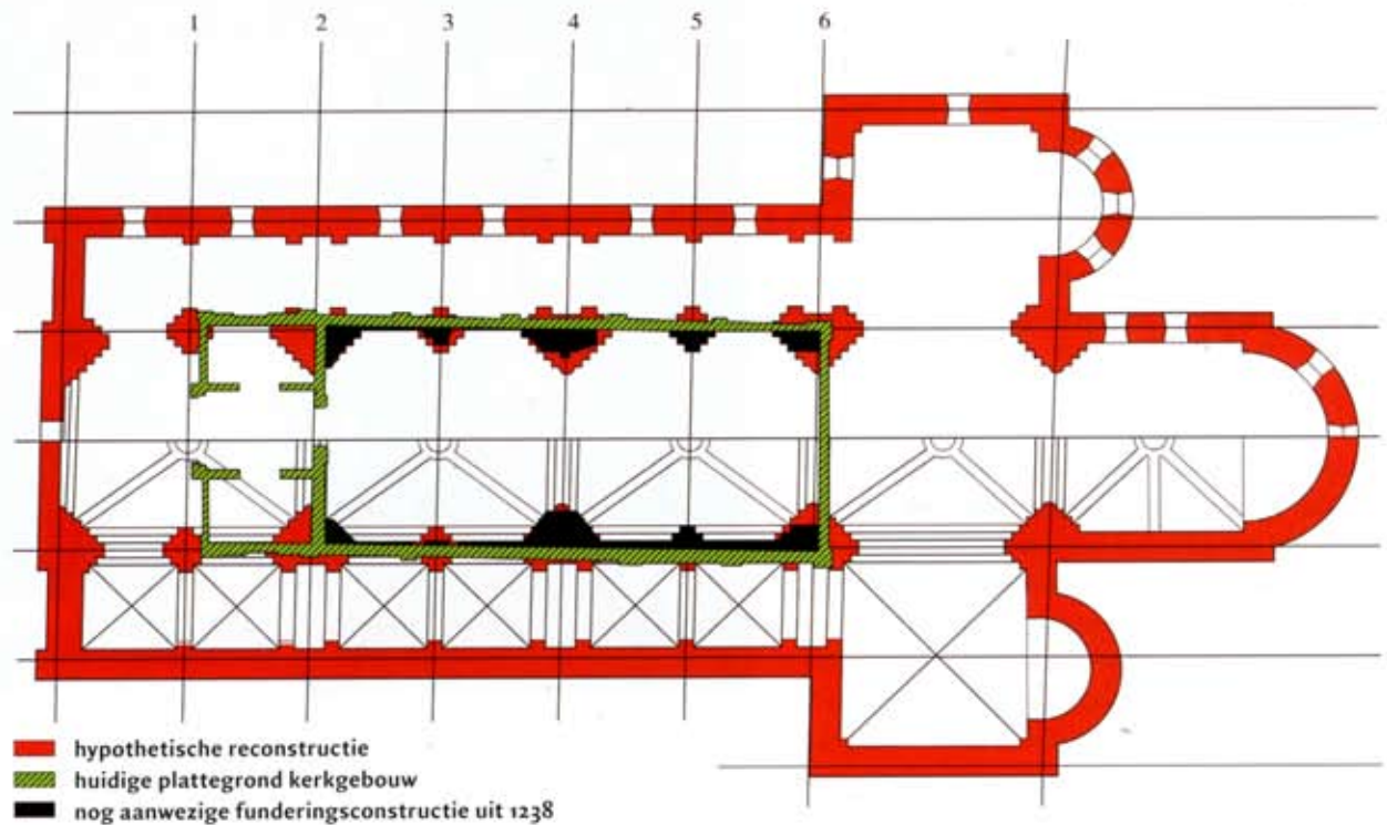
4 Reconstructie van de kloosterkerk door Battjes en Ladrak Bouwhistorici, Hoogezand/Erica
