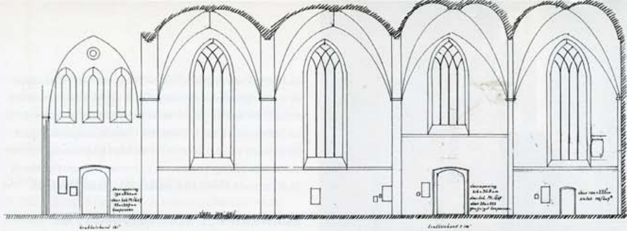
7 Martinikerk, zuidgevel van het schip, getekend in 1972 door J. Veldhuis tijdens de restauratie
