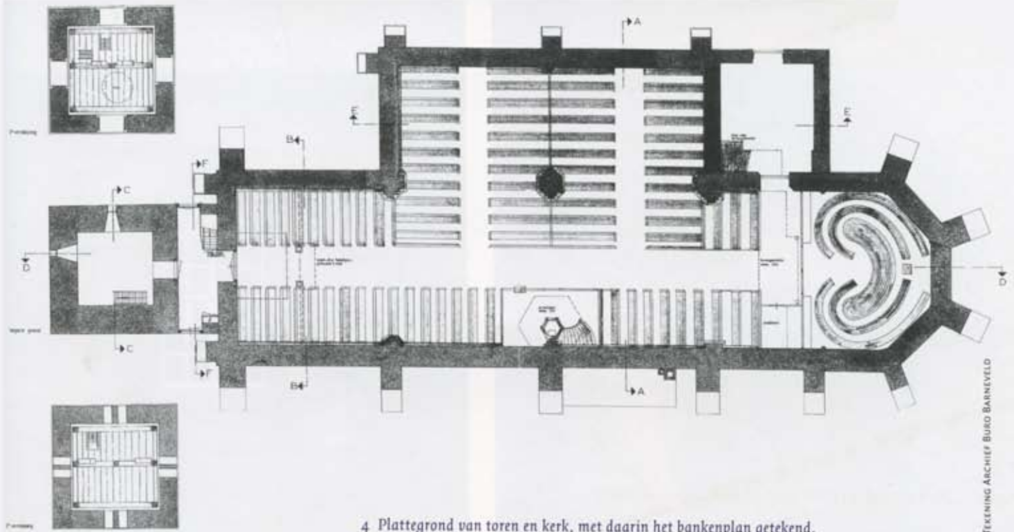
4 Plattegrond van toren en kerk, met daarin het bankenplan getekend. Tekening Architectenburo ir. P.B. Offringa, nu in archief OVT Architecten, Groningen.
